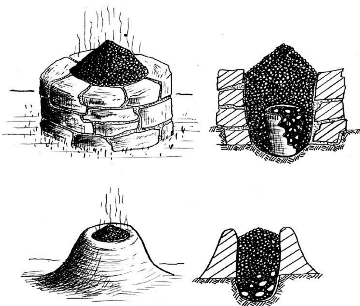
Медеплавильные горны
